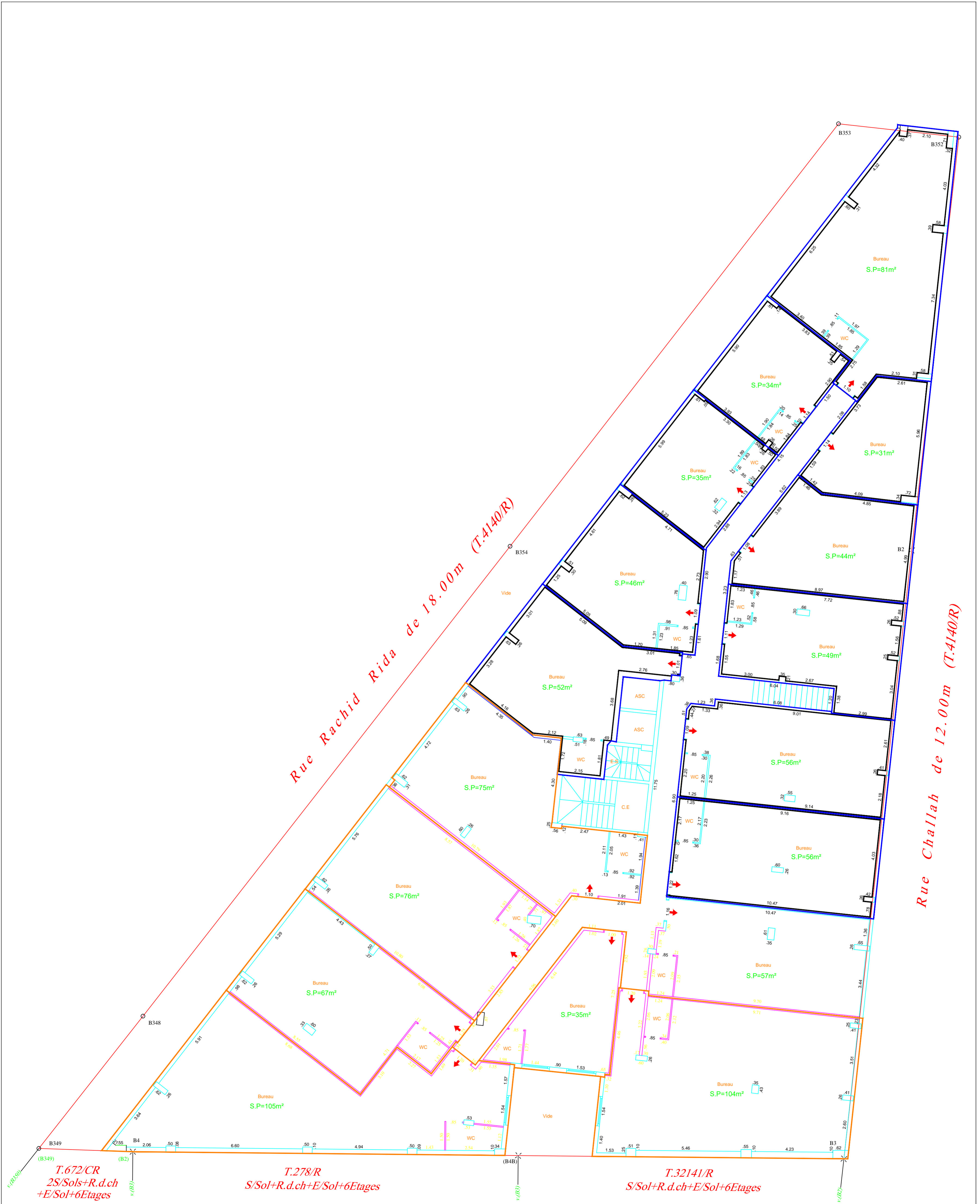
PLAN DE L'ENTRE SOL
